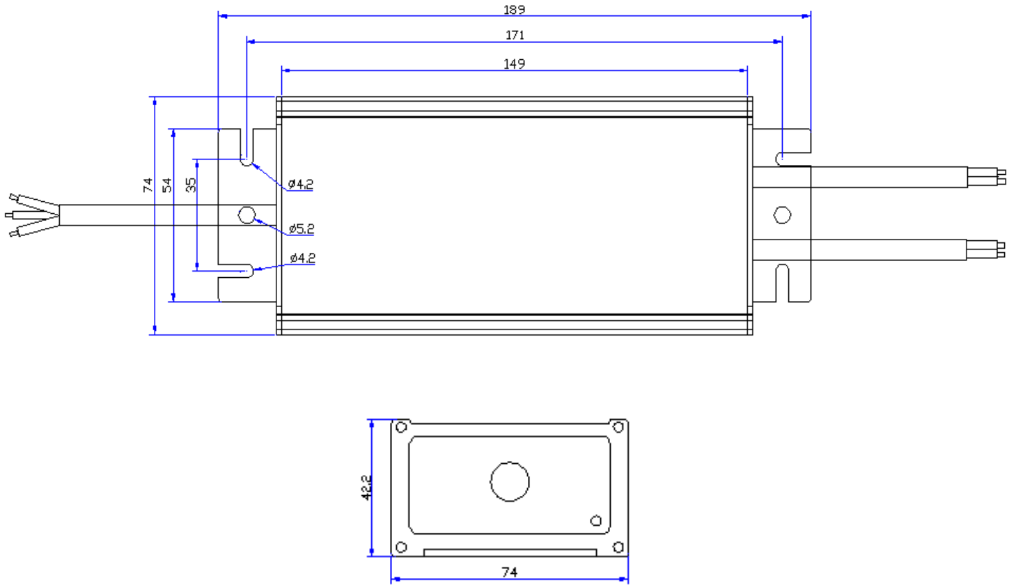
结构尺寸
